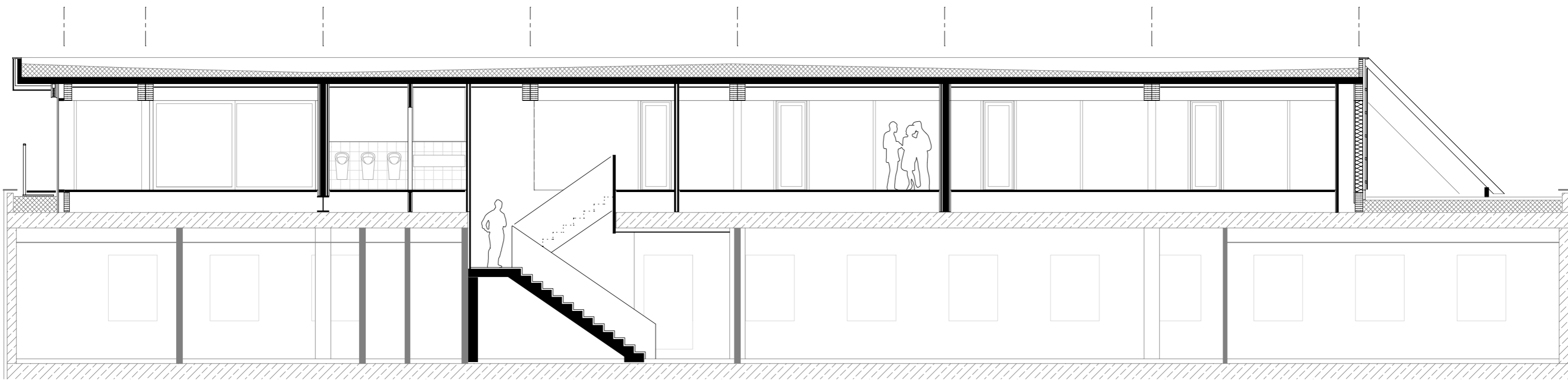
Längsschnitt M. 1:100
