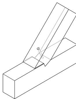
Heel notch joint
