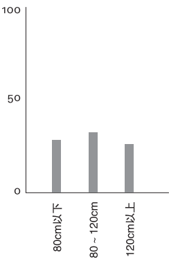
平均无缺陷工作长度比例， 以40/50mm宽度板材为例。
